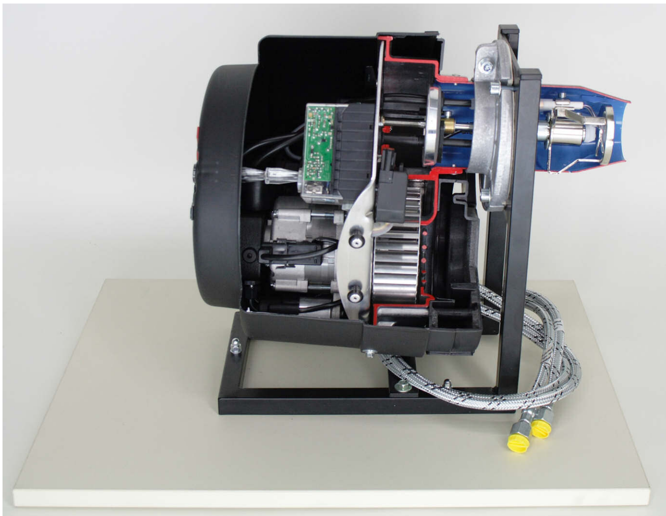
Abbildung zeigt Schnittmodell Ölbrenner Best-Nr. 0000 9610
